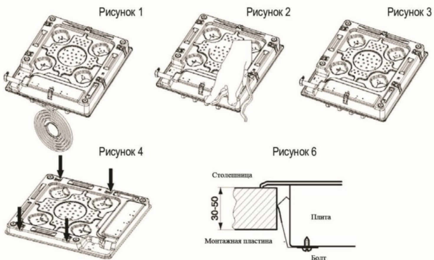
Точки установки монтажной пластины
